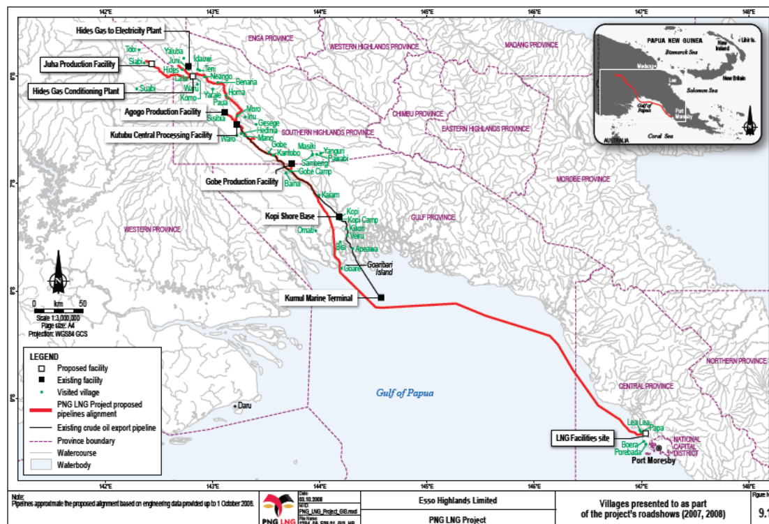
圖7. 巴布亞紐幾內亞液化天然氣計劃(出處：PNG LNG Project: Environmental Impact Statement Part I. 2009 January)
